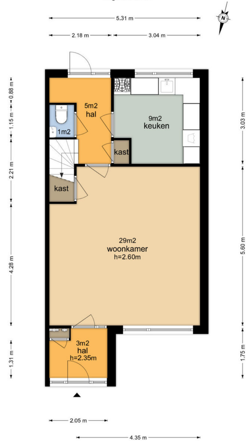
Benedictushof 87 - Vianen Begane Grond
