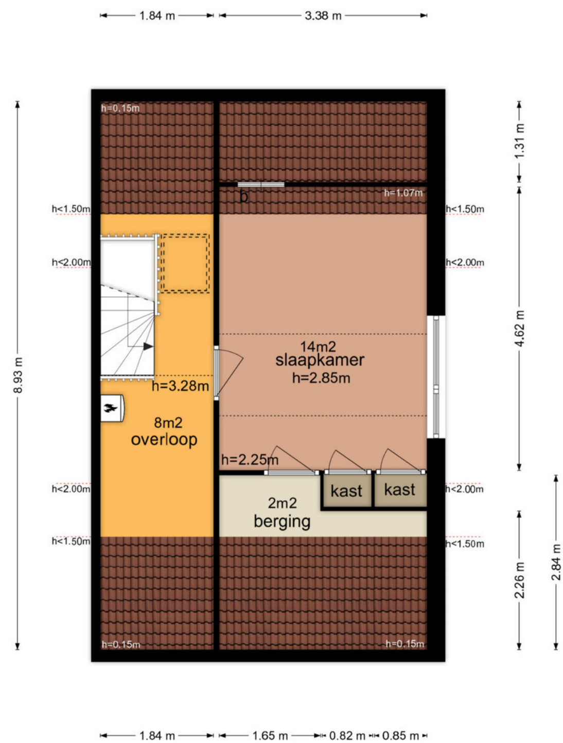
Benedictushof 87 - Vianen Tweede Verdieping
