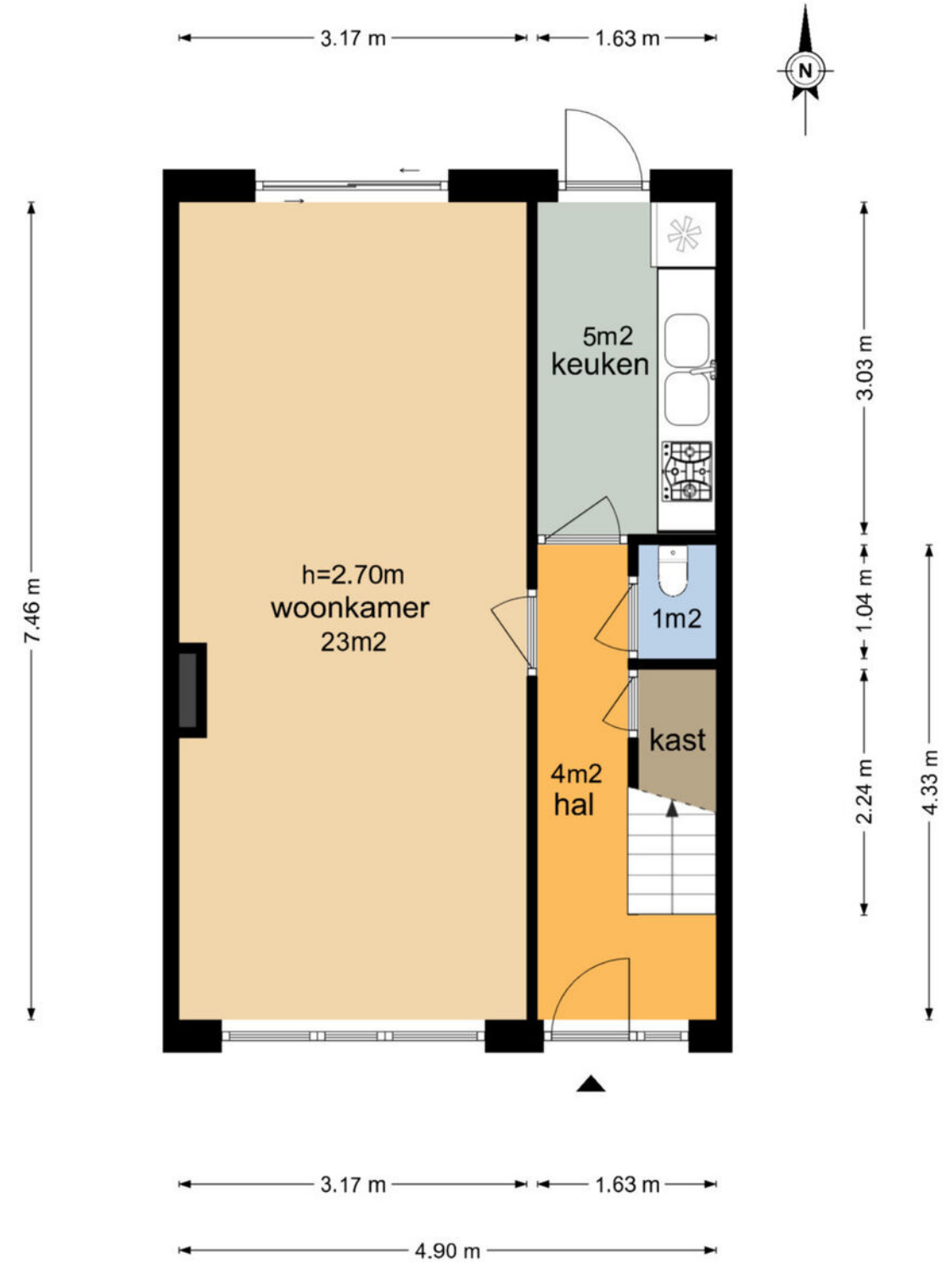
Hoendiepstraat 45 - Utrecht Begane Grond
