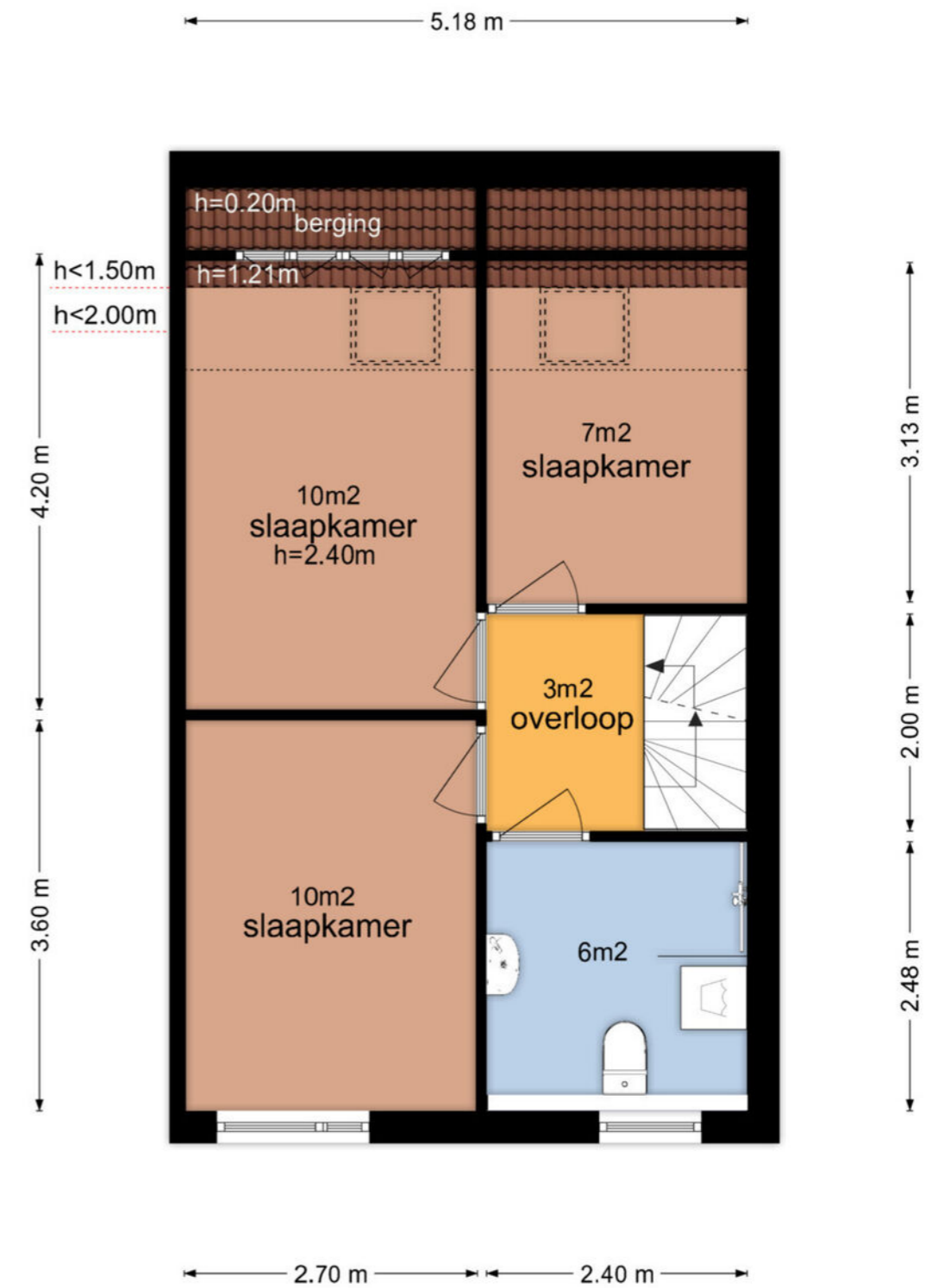
Graaf Dudosingel 9 - Nieuwegein Eerste Verdieping
