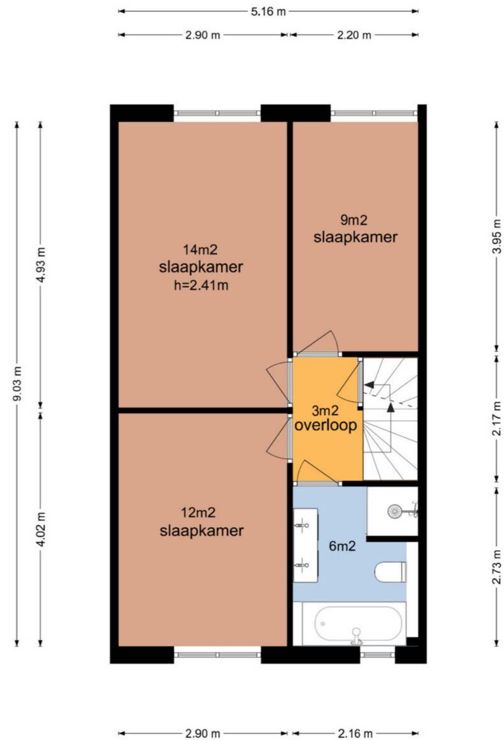
Graaf Rupertlaan 15 - Nieuwegein Eerste Verdieping
