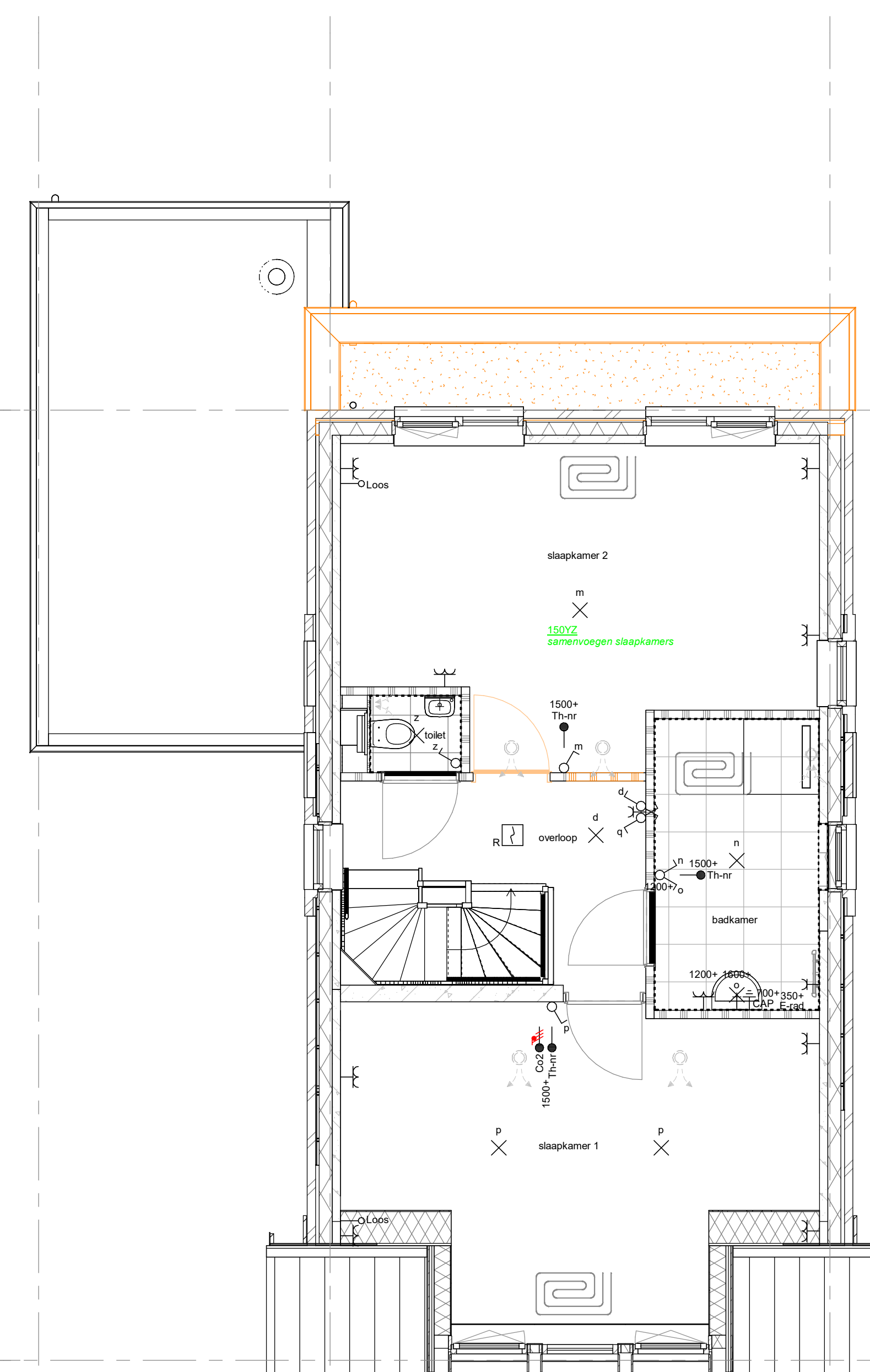
1e VERDIEPING
