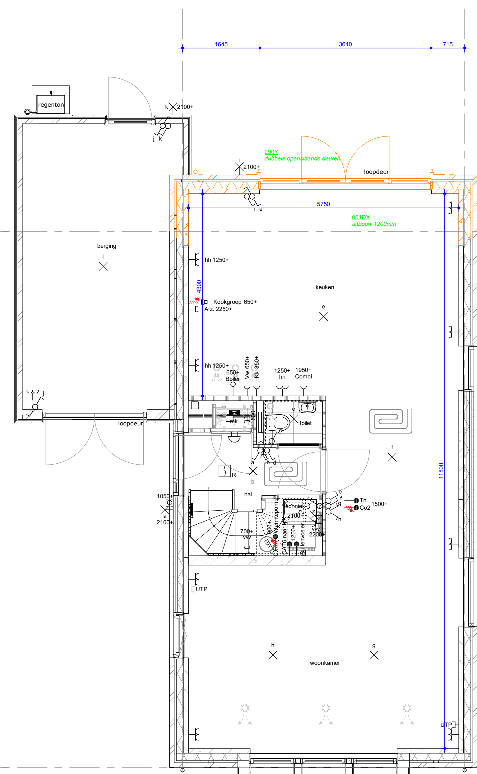
BEGANE GROND
