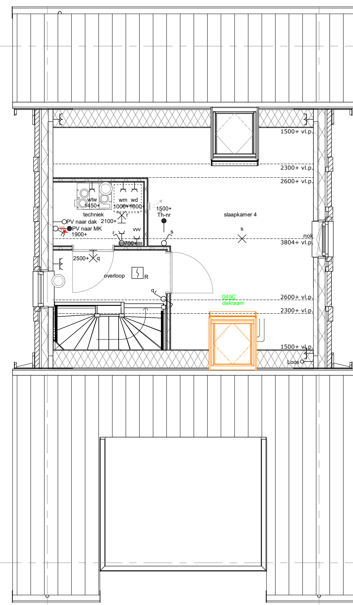
2e VERDIEPING
