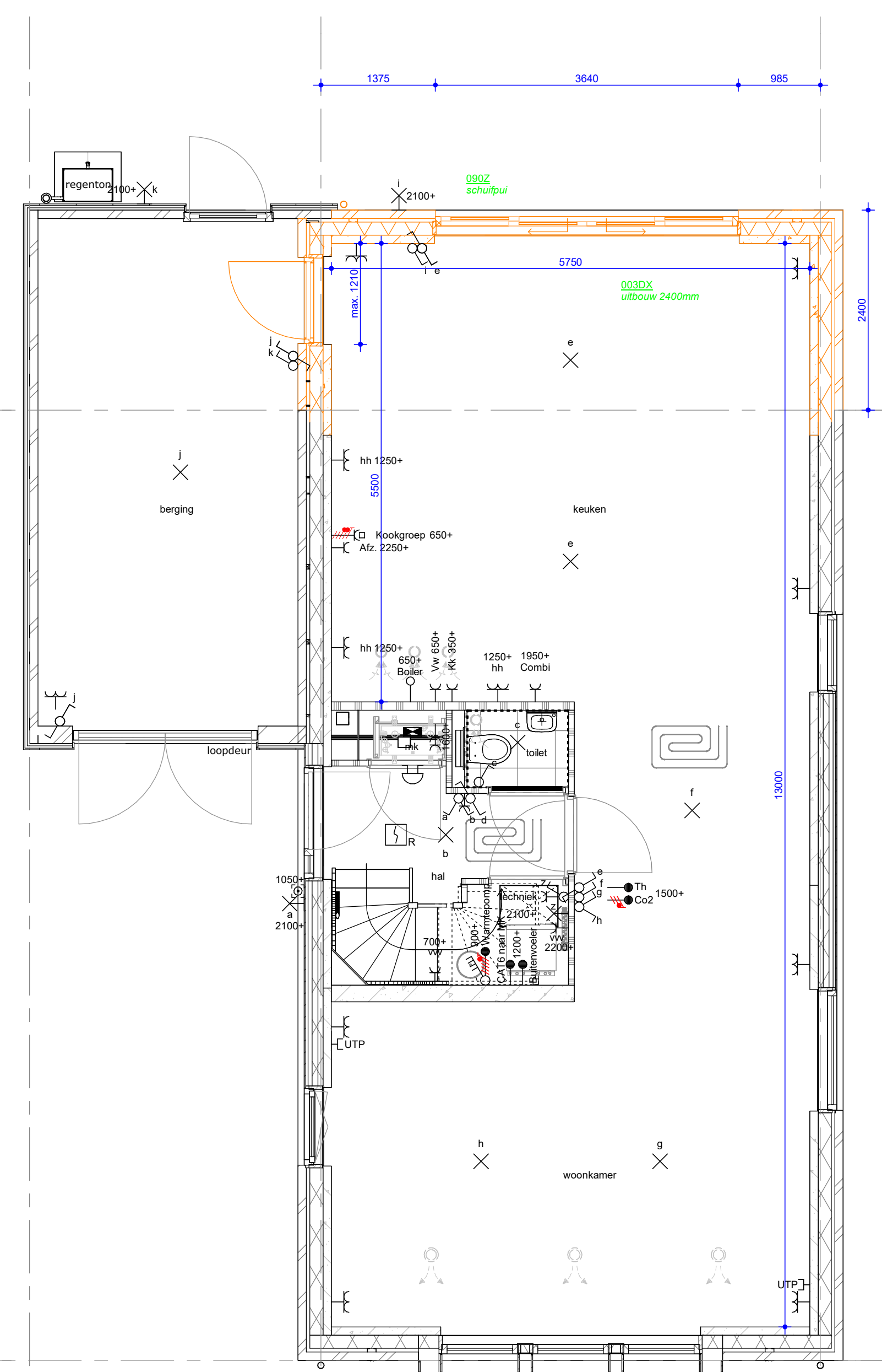
BEGANE GROND
