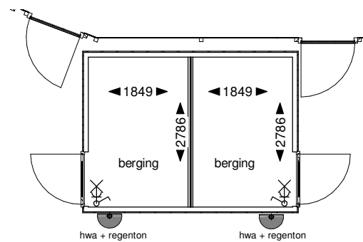
Begane grond
