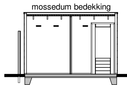
Doorsnede A
