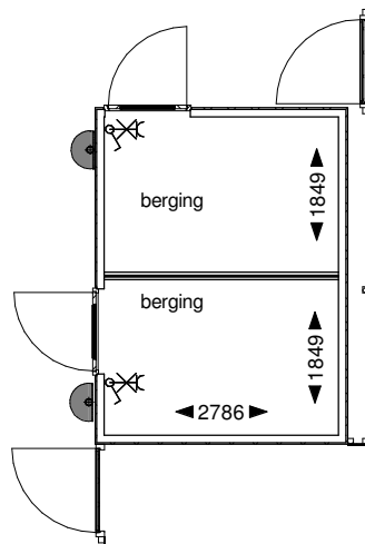
Begane grond
