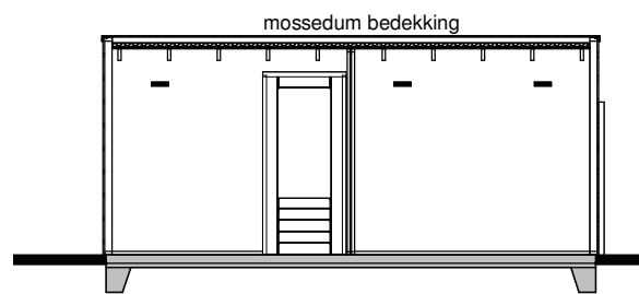
Doorsnede A
